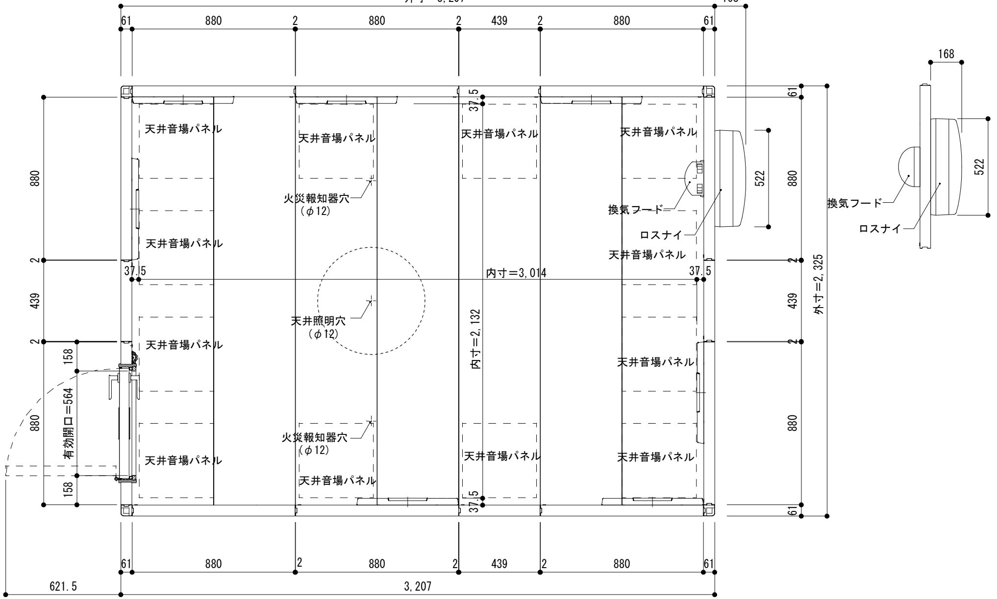
4.3畳 平面図 S=1/20
